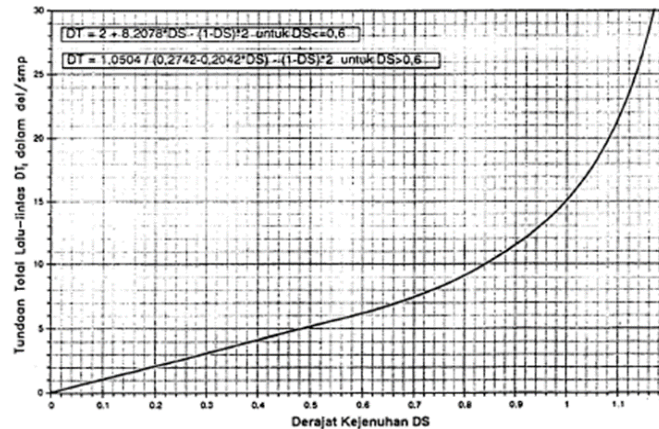
Gambar 1. Tundaan Lalu Lintas Simpang ( DT_1 ) Sumber: MKJI (1997)
