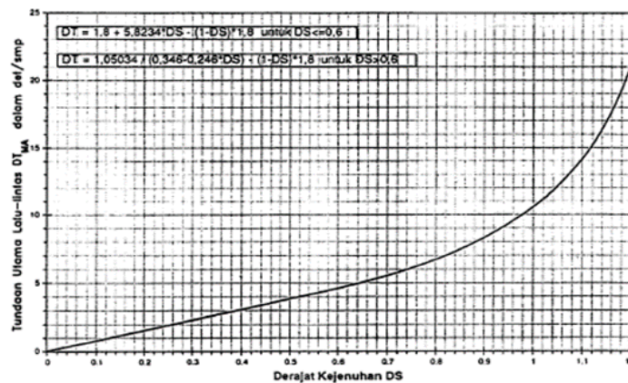
Gambar 2. Tundaan Lalu Lintas Jalan Utama ( DT_{MA} ) Sumber: Departemen PU, 1997
