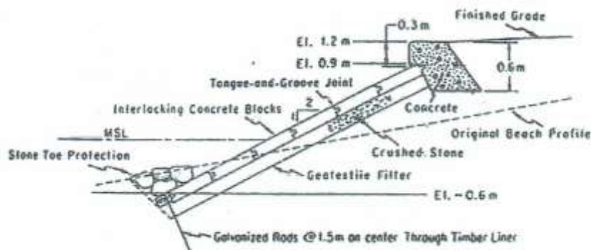
Gambar 2. Revetment dengan Interlocking Concrete-Block (Triatmodjo, 1999)
