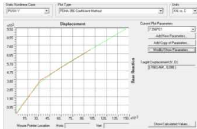
Gambar 9. Kurva koefisien perpindahan FEMA 356 arah Y
