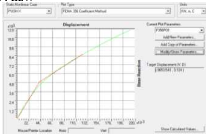
Gambar 8. Kurva koefisien perpindahan FEMA 356 arah X
