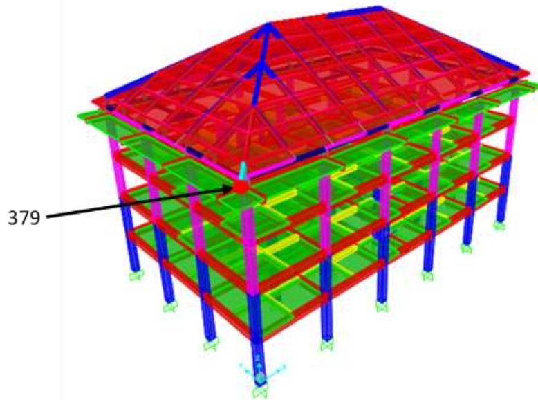
Gambar 2. Pemodelan 3D SAP2000
