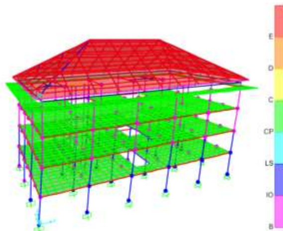
Gambar 3. Penyebaran sendi plastis
